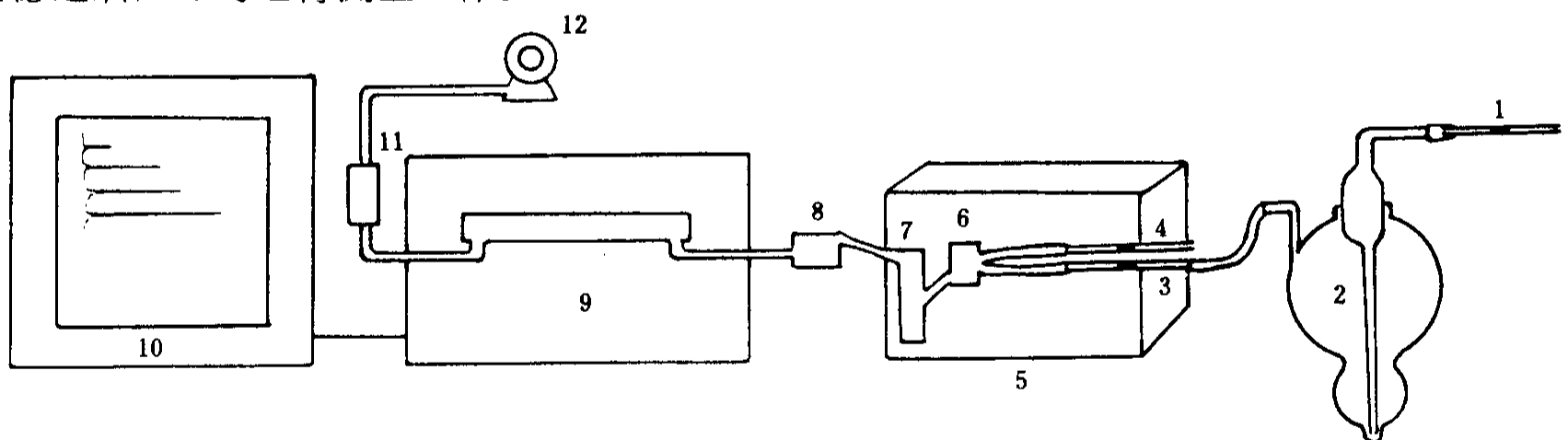
汞蒸气测定的气路流程
